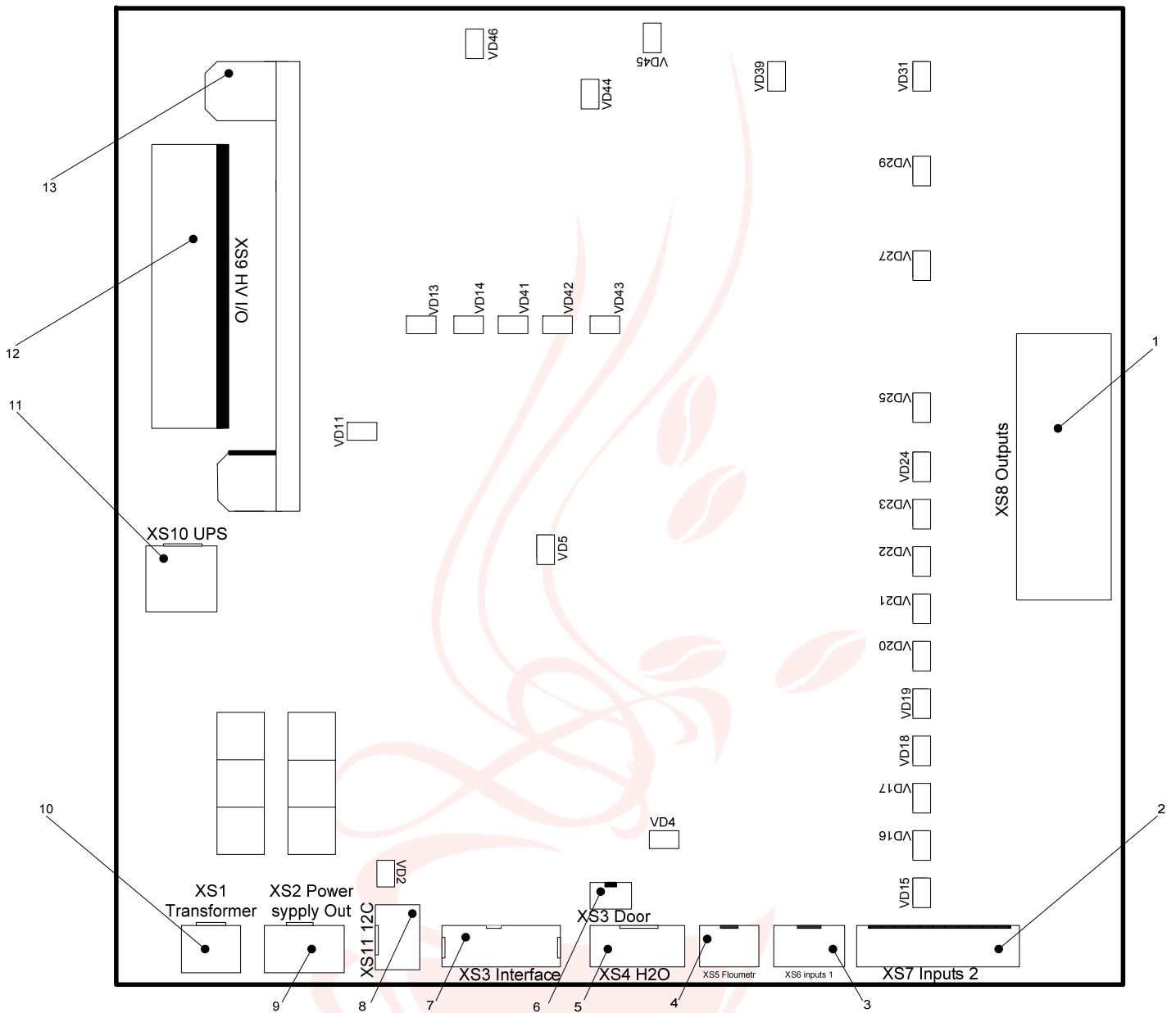
Рис. 7. Плата автоматики
