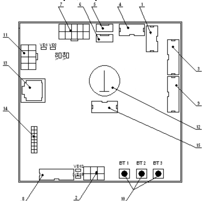
Рис. 8. Процессорная плата
