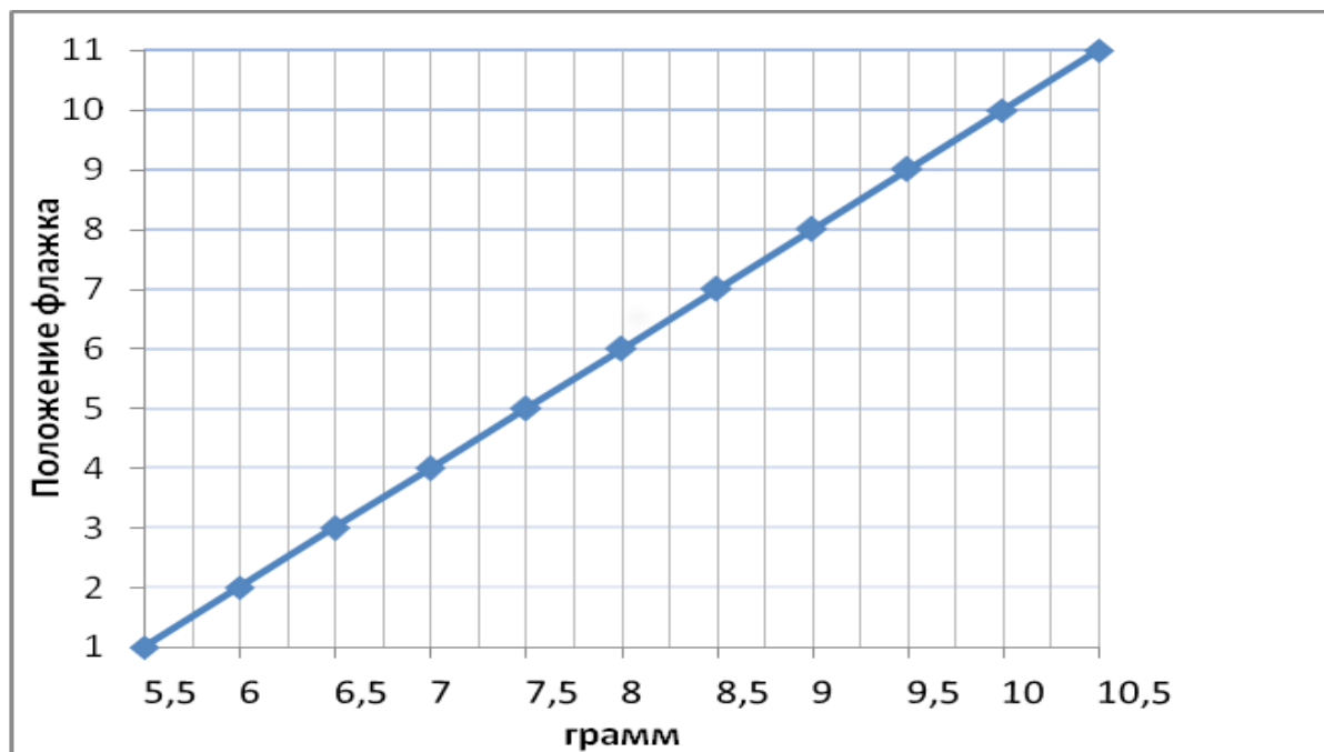
Рис. 12. График зависимости дозировки натурального кофе.
