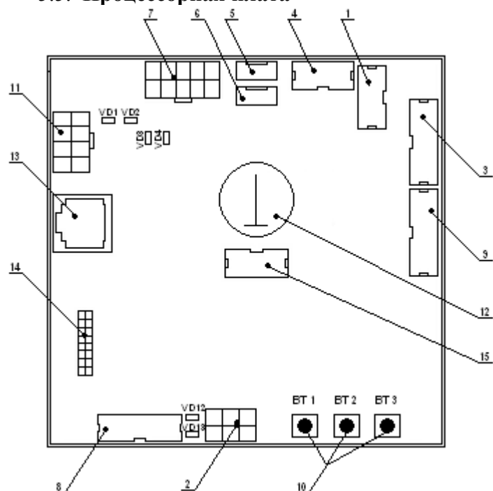
Рис. 8. Процессорная плата
