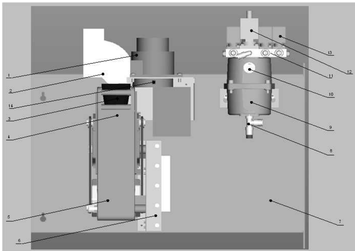
Рис. 5. Блок приготовления заварного кофе.
