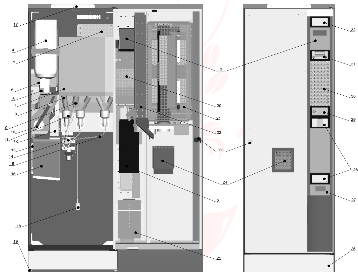
Рис 1. Составные части торгового автомата МК - 01
