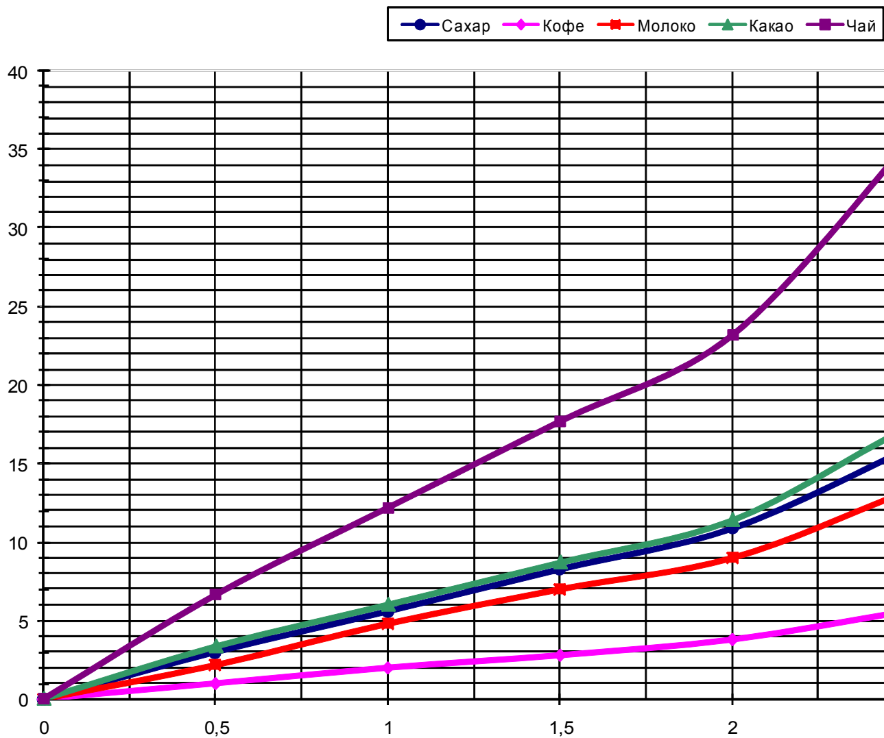
Рис 11. График зависимости времени (вращения шнека) и позиций дозатора от количества выдаваемого ингредиента
