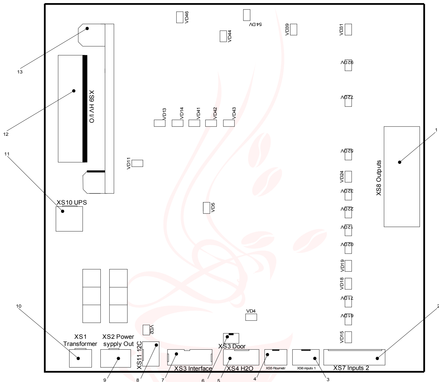
Рис. 7. Плата автоматики
