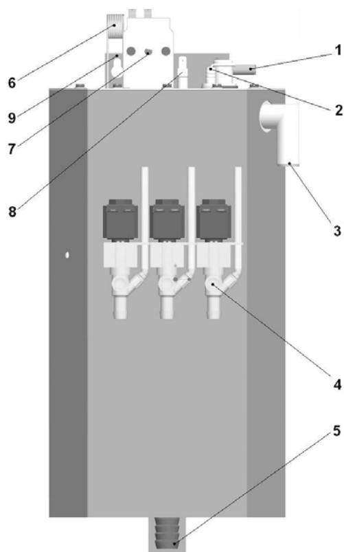
Рис. 5. Бойлер
